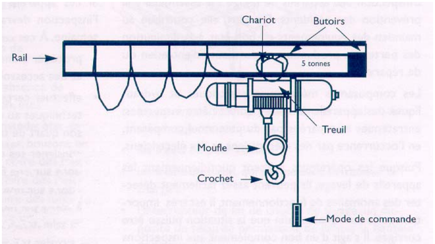
Composantes d'un palan motorisé
