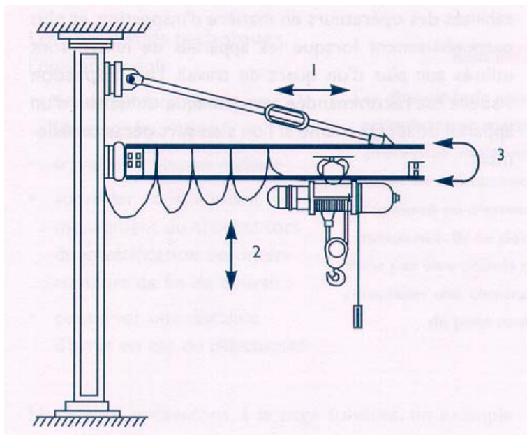
Composantes d'un palan motorisé
